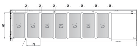
KONFIGURACJA 7×GN1/3
