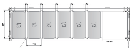
KONFIGURACJA 6×GN1/3
